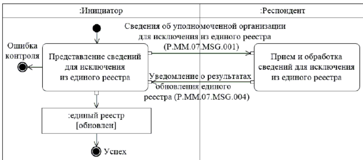
Рис. 6. Схема выполнения транзакции общего процесса "Передача сведений об уполномоченной организации для исключения из единого реестра" (P.MM.07.TRN.003)
